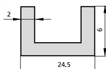
TÊTIÈRE U
