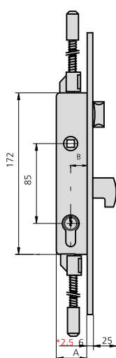
TÊTIÈRE U
