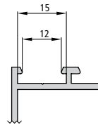
CE202/6LR20 Inox. central regulable para serie 202-302
