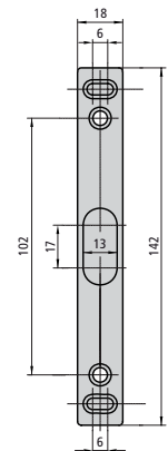
CE202S/6LR18 Inox. alto/bajo regulable para serie 202
