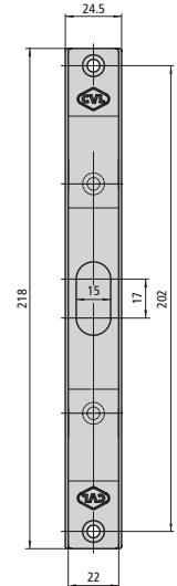
CE202S/1NRS Metálico pintado en negro alto/bajo regulable para serie 202
