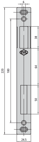
CE202/6LAN Inox. central para serie 202-302
