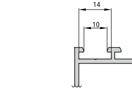
CE202/6LR18 Inox. central regulable para serie 202-302
