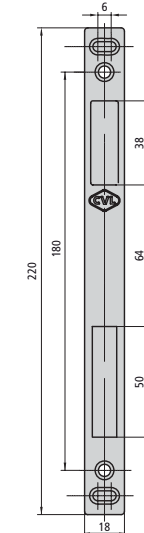
CE202/6LR18 Inox. central regulable para serie 202-302
