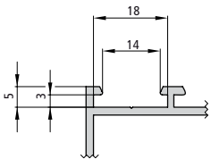
CE202/1NR Metálico pintado en negro central regulable para serie 202-302
