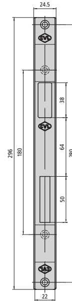
CE202/1NRS Metálico pintado en negro central regulable para serie 202-302
