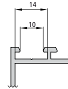
CE202S/6LR18 Inox. alto/bajo regulable para serie 202
