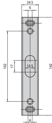
CE202S/6U Inox. alto/bajo en U para serie 202
