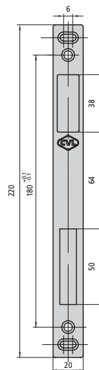
CE202/6LR20 Inox. central regulable para serie 202-302
