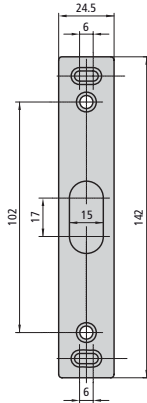
CE202S/6LAN Inox. alto/bajo para serie 202
