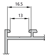
CE202S/1NR Metálico pintado en negro alto/bajo regulable para serie 202
