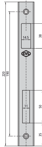
CE202/6U Inox. central en U para serie 202-302
